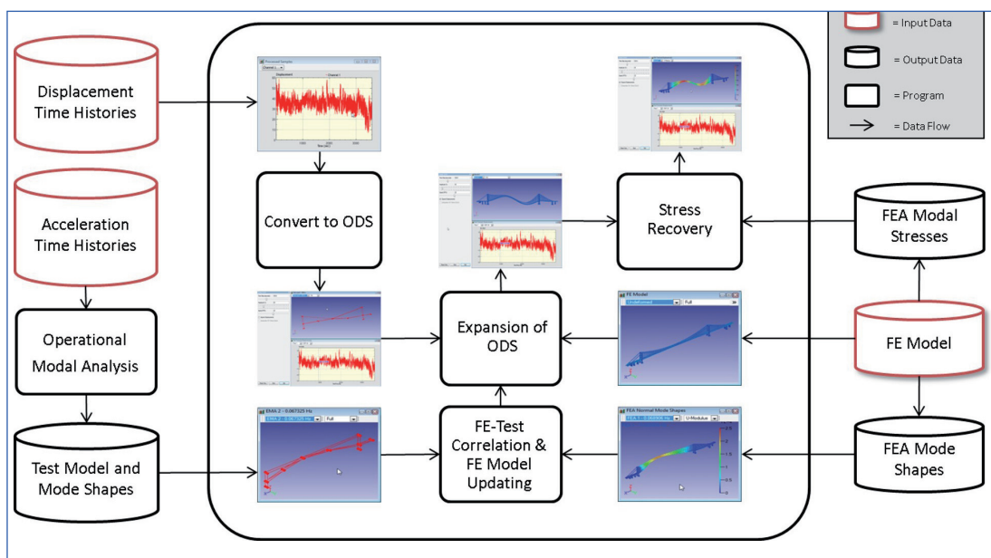
Figura 1 – Flowchart del metodo ibrido numerico-sperimentale
